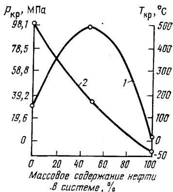
Рис. 3.27. Зависимость критических давлений p_{кр} (1) и температуры T_{кр} (2) системы нефть — конденсатный газ от содержания в ней нефти. Степновское месторождение (пласт D 2 IV a , плотность нефти 859 кг/м 3 , содержание конденсата в газе 51 г/м 3 , плотность конденсата 736 кг/м 3 , относительная плотность газа без конденсата 0,621)
