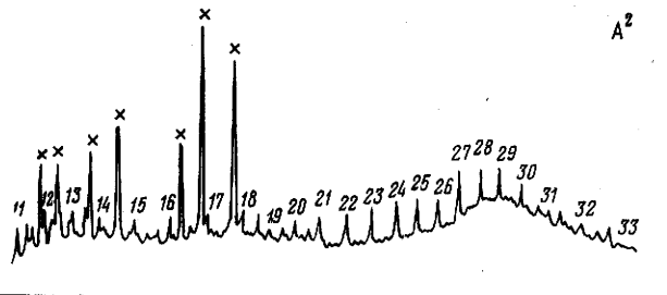
Рис. 2.4. Хроматограммы ароматических УВ (Л. В. Колесникова, 1971 г.) 1 — бензол; 2 — толуол; 3 — этилбензол; 4 — м -ксилол; 5 — п -ксилол; 6 — изопропилбензол; 7 — о -ксилол; 8 — н -пропилбензол; 9 — 1-метил-3-этилбензол; 10 — 1-метил-4-этилбензол; 11 — 1,3,5-триметилбензол; 12 — изобутилбензол; 13 — 1-метил-2-этилбензол; 14 — м -цимол; 15 — п -цимол; 16 — 1,2,4-триметилбензол; 17 — 1-метил-4- н -пропилбензол; 18 — 1-метил-3- н -пропилбензол; 19 — не идентифицирован; 20 — н -бутилбензол; 21 — 1,2-диэтилбензол; 22 — не идентифицирован; 23 — 1,2,3-триметилбензол
