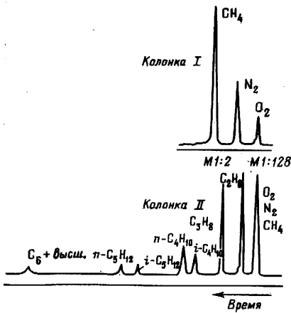
Рис. 2.1. Хроматограммы газов (В. Ф. Камьянов, 1970 г.)
