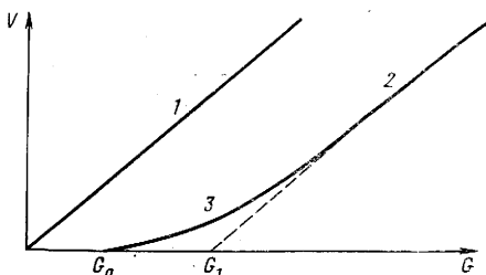
Рис. 9.1. Зависимость скорости фильтрации v от напорного градиента G .
