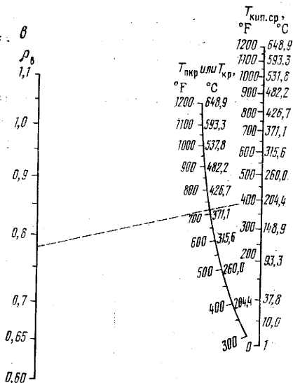
Рис. 3.20. Номограммы для определения в углеводородных смесях псевдокритического \rho_{\text{кр}} (а) и критического \rho_{\text{кр}} (б) давления, критической T_{\text{кр}} и псевдокритической T_{\text{кр}} температуры (в) [74]. T_{\text{кип. ср}} — температура средняя молярная для T_{\text{кр}} и средняя массовая для T_{\text{кр}}
