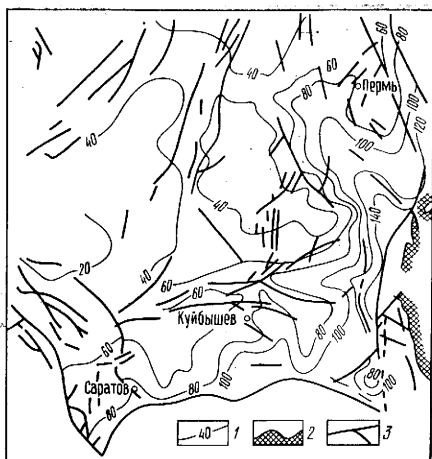
Рис. 6.6. Карта геоизотерм поверхности кристаллического фундамента Волго-Уральской нефтегазоносной провинции (А. В. Дружинин, 1969 г.). 1 — изотермы, °С; 2 — граница Восточно-Европейской платформы; 3 — разломы
