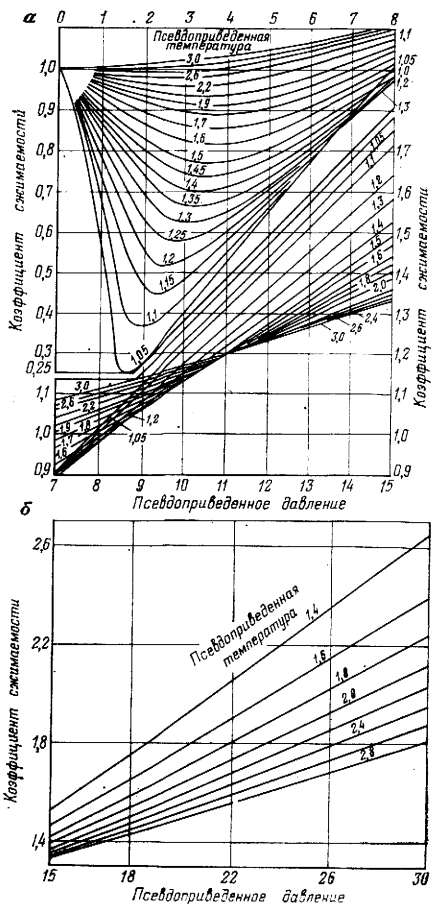
Рис. 3.1. Псевдокритические свойства природных газов [54].
