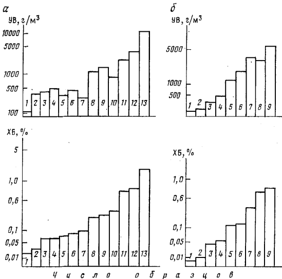
Рис. 2.17. Диаграммы зависимости между содержанием в породах битумида ХВ и УВ (основной части микро нефти). Коэффициент ранговой корреляции (по К. Спирмену) для пород:
