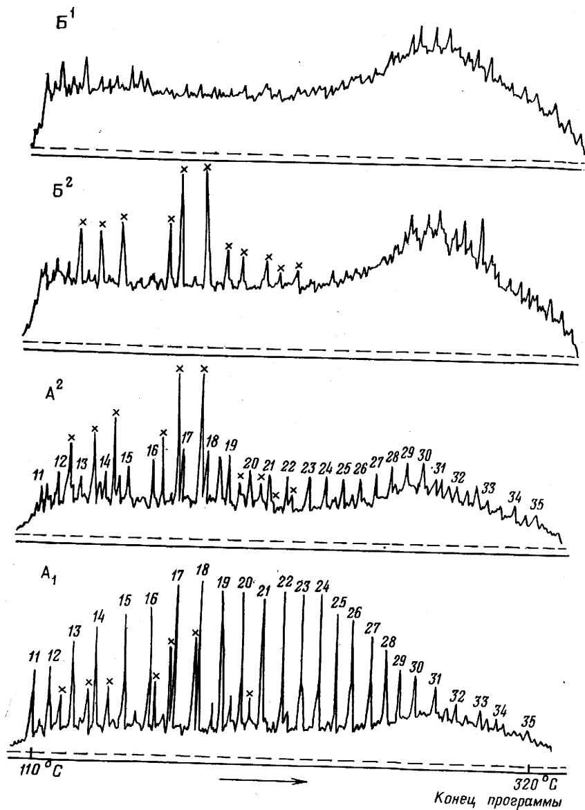
Рис. 2.9. Хроматограммы нефтей различных химических типов (средние данные по 300 нефтям месторождений СССР). По Ал. А. Петрову.
