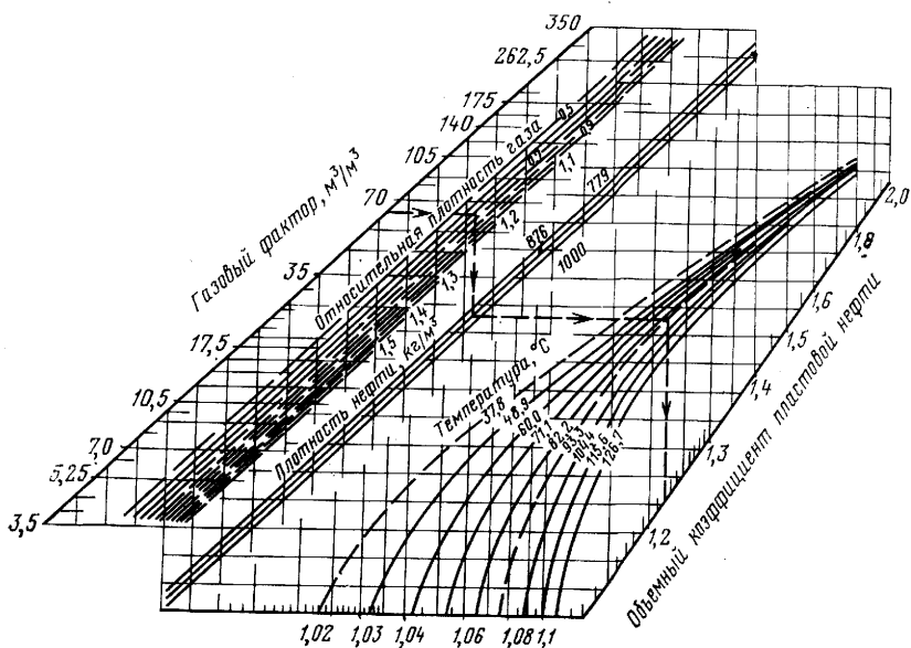
Рис. 3.13. Номограмма для определения объемного коэффициента пластовой нефти [54]
