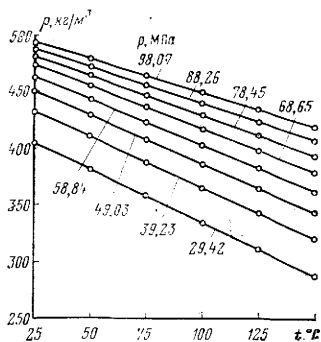
Рис. 3.35. Зависимость плотности \rho системы метан — n -гексан ( N_2 0,2) от температуры t при разном давлении (А. В. Сушилиин, Г. П. Сафронова, Т. П. Жузе, 1973 г.)
