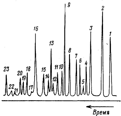
Рис. 2.4. Хроматограммы ароматических УВ (Л. В. Колесникова, 1971 г.) 1 — бензол; 2 — толуол; 3 — этилбензол; 4 — м -ксилол; 5 — п -ксилол; 6 — изопропилбензол; 7 — о -ксилол; 8 — н -пропилбензол; 9 — 1-метил-3-этилбензол; 10 — 1-метил-4-этилбензол; 11 — 1,3,5-триметилбензол; 12 — изобутилбензол; 13 — 1-метил-2-этилбензол; 14 — м -цимол; 15 — п -цимол; 16 — 1,2,4-триметилбензол; 17 — 1-метил-4- н -пропилбензол; 18 — 1-метил-3- н -пропилбензол; 19 — не идентифицирован; 20 — н -бутилбензол; 21 — 1,2-диэтилбензол; 22 — не идентифицирован; 23 — 1,2,3-триметилбензол
