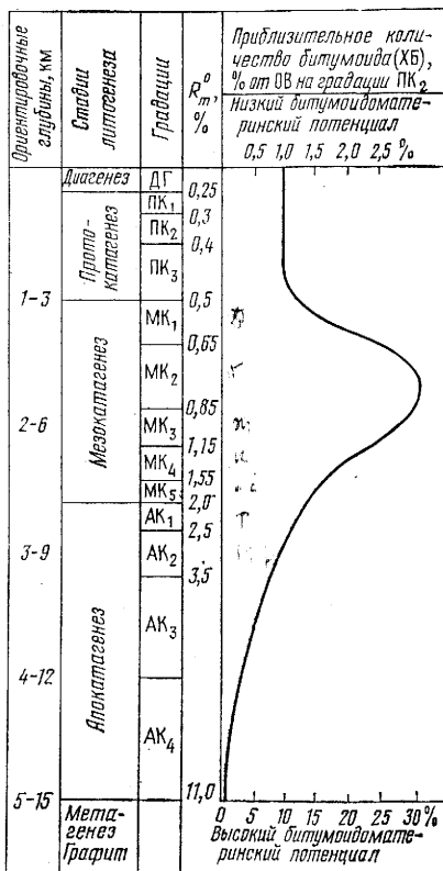
Рис. 2.14. Ориентировочная схема изменения в процессе катагенеза коэффициента \beta_{XB} , т. е. содержания битумоида в ОБ.
