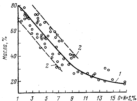
Рис. 2.13. Зависимость между содержанием масел и количеством гетероэлементов в хлороформном битумоиде глин Западно-Кубанского прогиба. По Ю. И. Корчагиной, 1974 г. 1 — кривая среднего содержания масел и гетероэлементов; 2 — границы отклонений
