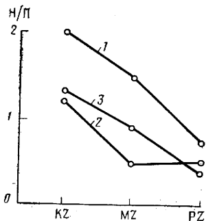
Рис. 8.8. Зависимость величины отношения содержаний нафтеновых и парафиновых УВ (H/П) для нефтей и бензинов от возраста вмещающих отложений (А. А. Карцев, 1960 г.). 1 — нефти; 2 — бензины; 3 — легкие бензины
