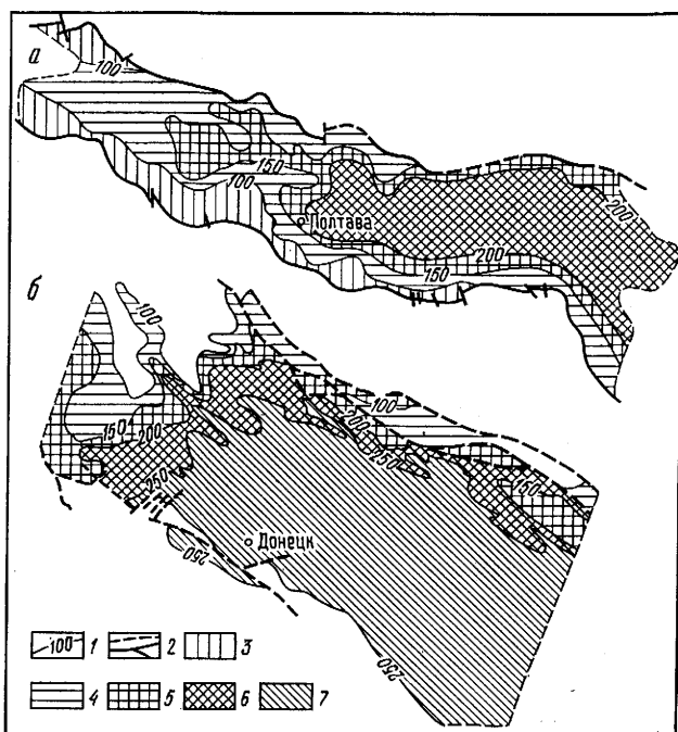
Рис. 6.15. Схема распределения палеотемпературы в кровле вблизи Днепровско-Донецкой впадины по Н. П. Гречишникову и В. Н. Летуновскому (а) и на поверхности карбона в Донбассе по И. И. Аммосову (б).
