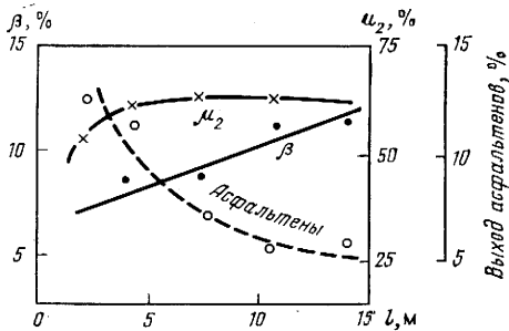
Рис. 2.18. Зависимость содержания битуминов (фиксируемого величины \beta ) и их состава (количество УВ — M_2 и асфальтенов) в нефтематеринском ОБ девонских аргиллитов от расстояния до коллектора 1 (Восточная Сахара, Алжир)
